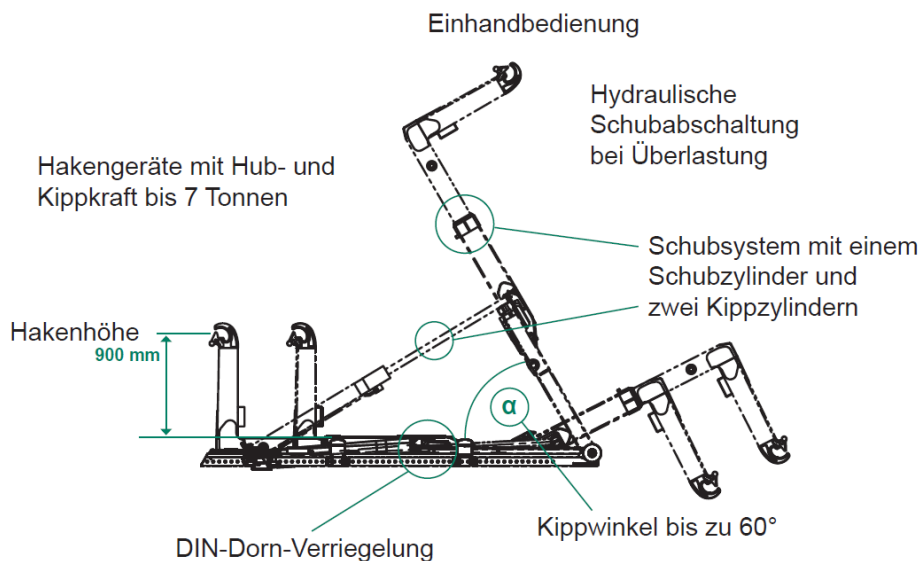
Abbildung: UNSINN Abrollsystem nach DIN 30722 Teil 3
